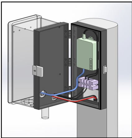
ELSEEVEとの設置イメージ図 (端子台あり)
