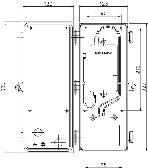
製品寸法 (端子台なし)
